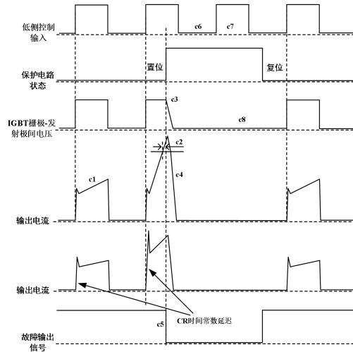
图 12 短路电流保护时序图（只适合于低侧）
