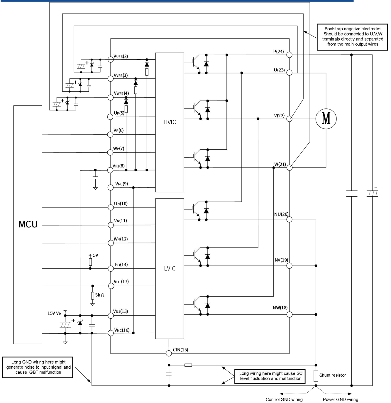
图16 典型应用电路
