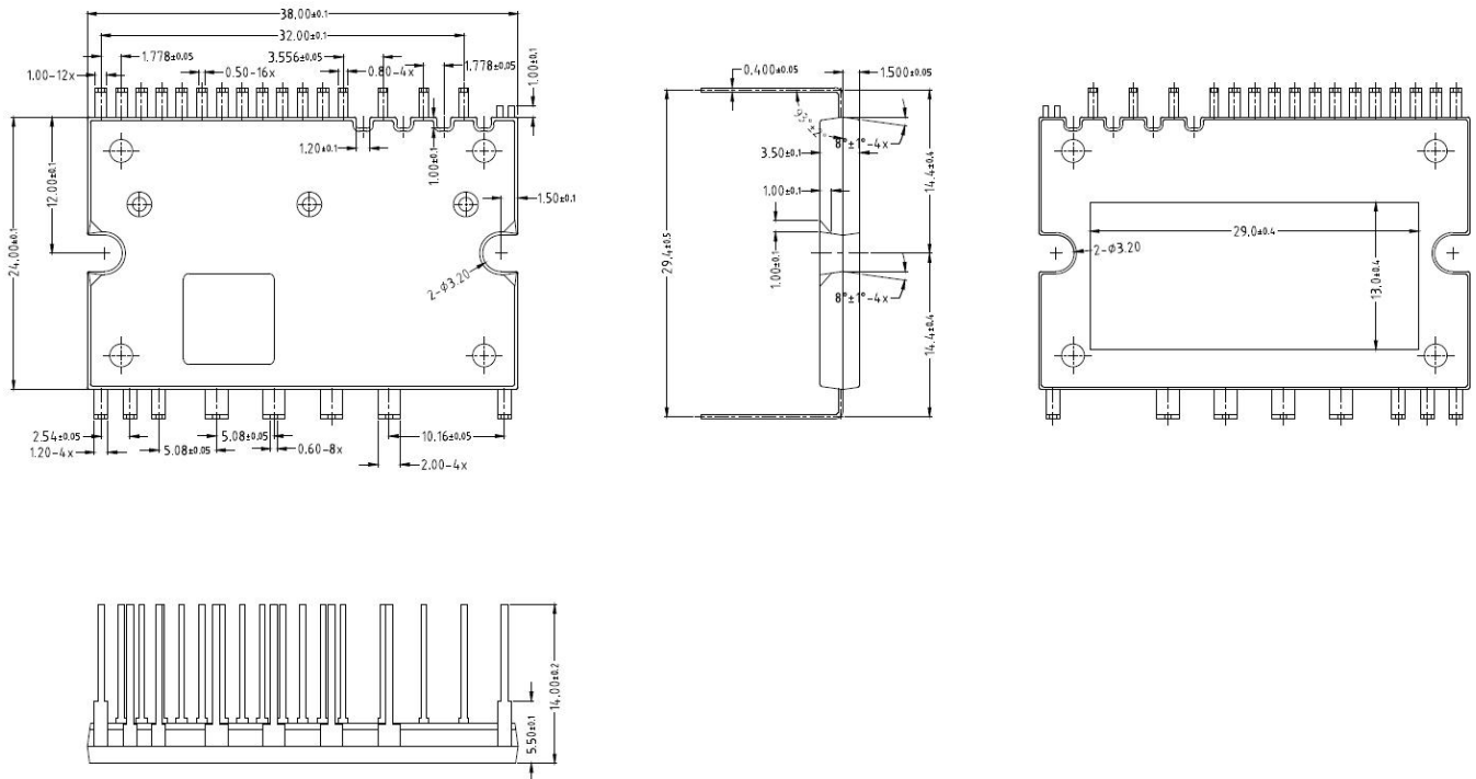
图17 外型封装图
