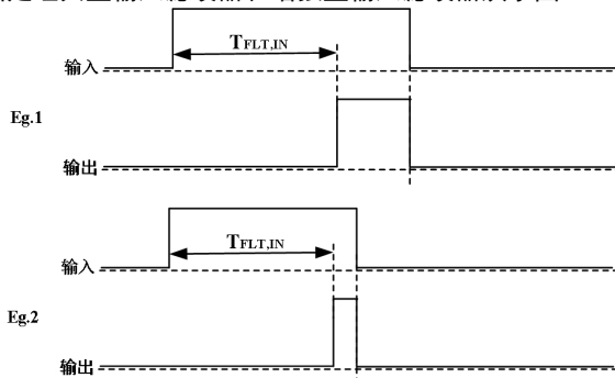
图 8 典型输入滤波
