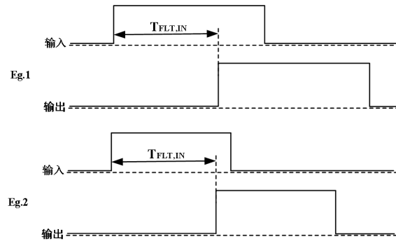
图 9 增强型输入滤波
